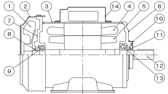
ภาพที่ 6: ส่วนประกอบมอเตอร์
