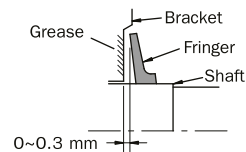
ภาพที่ 9: การประกอบ Fringer และระยะประกอบ
