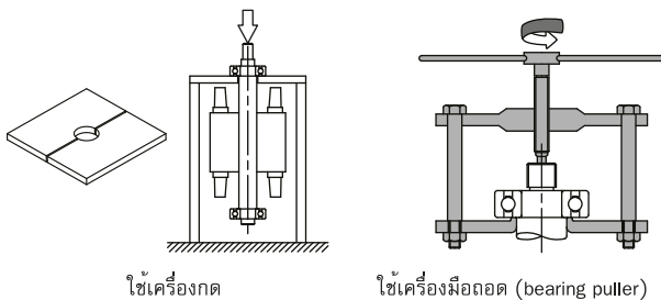
ภาพที่ 13: การถอดตลับลูกปืนออกจากเฟลา โดยใช้เครื่องกด และเครื่องมือถอด
